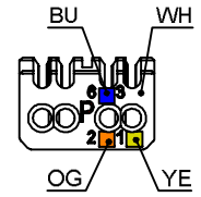
Anschlussbelegung / PIN assignment Profinet / industrial
