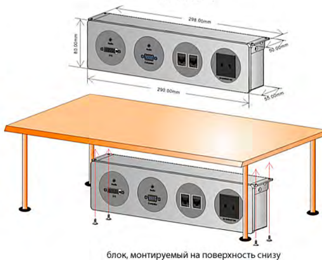
ТВ-RMU-4
