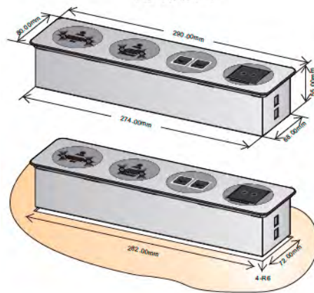
ТВ-RMM-4
