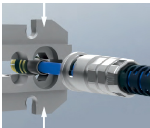
3. Обожмите экран и внешнюю оболочку кабеля втулкой
