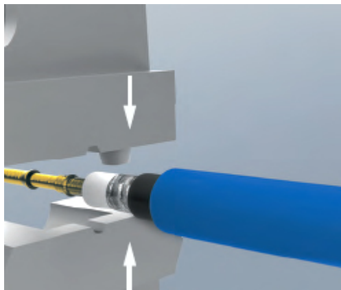
1. Обожмите центральный контакт
