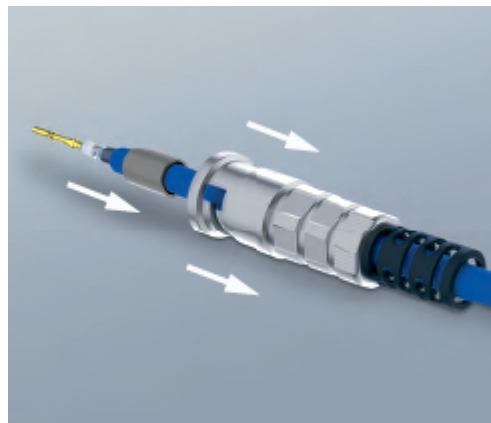
2. Наденьте на кабель корпус с хвостовиком
